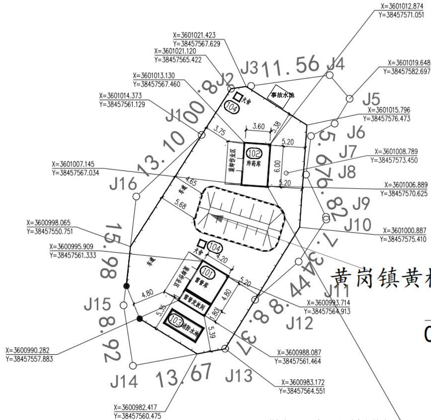
附图二 项目平面布置图-2
