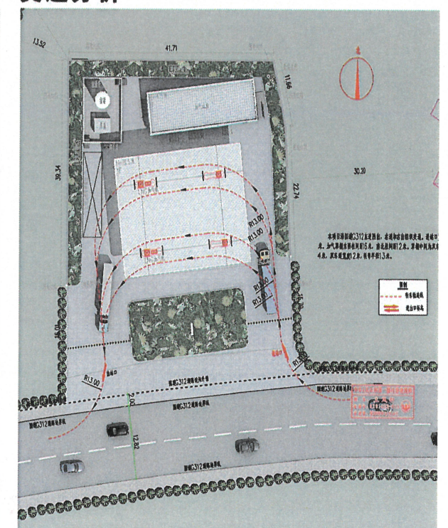
交通分析
