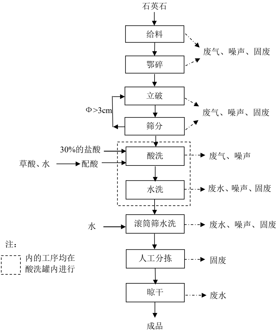
图 2-5 项目营运期生产工艺及产污环节示意图
