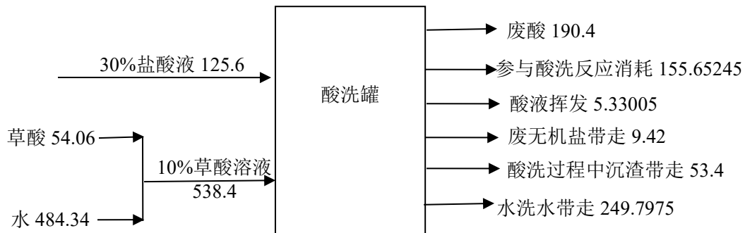
图 2-3 本项目酸液物料平衡图 单位 t/a
