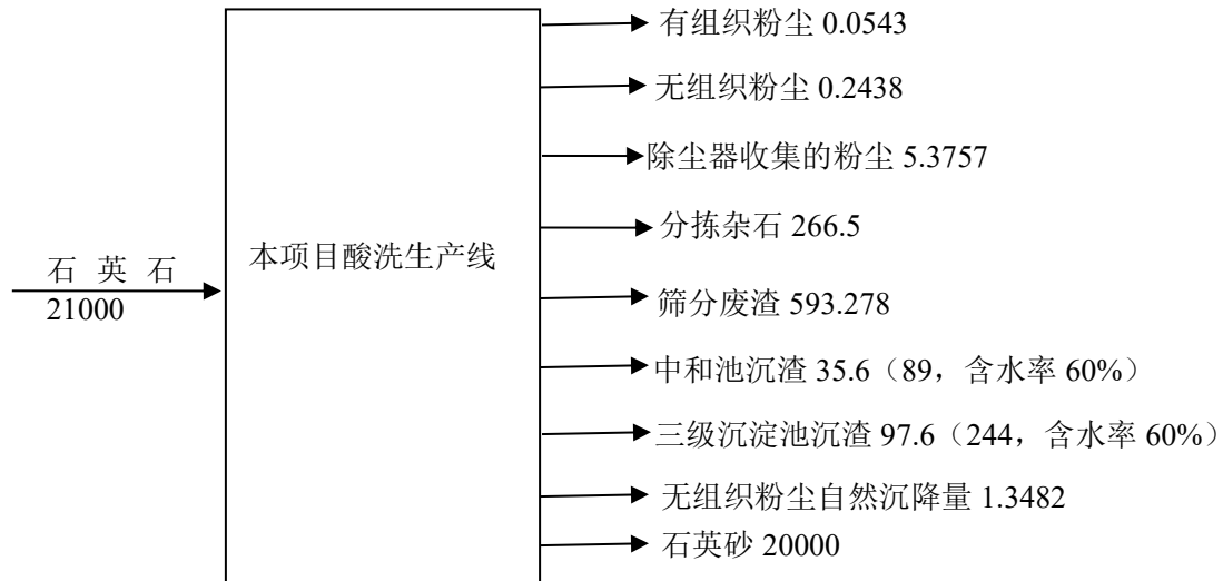
图 2-2 本项目石英石物料平衡图 单位 t/a
