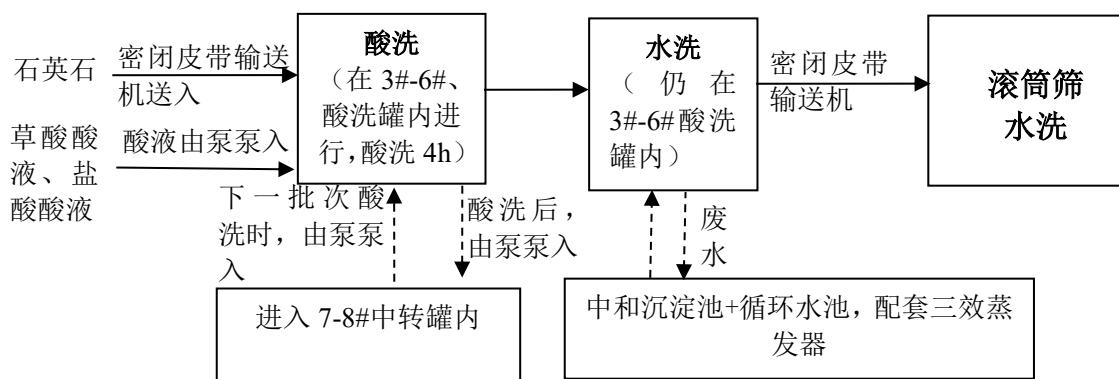
图 2-6 项目酸洗、水洗全过程工艺流程图
