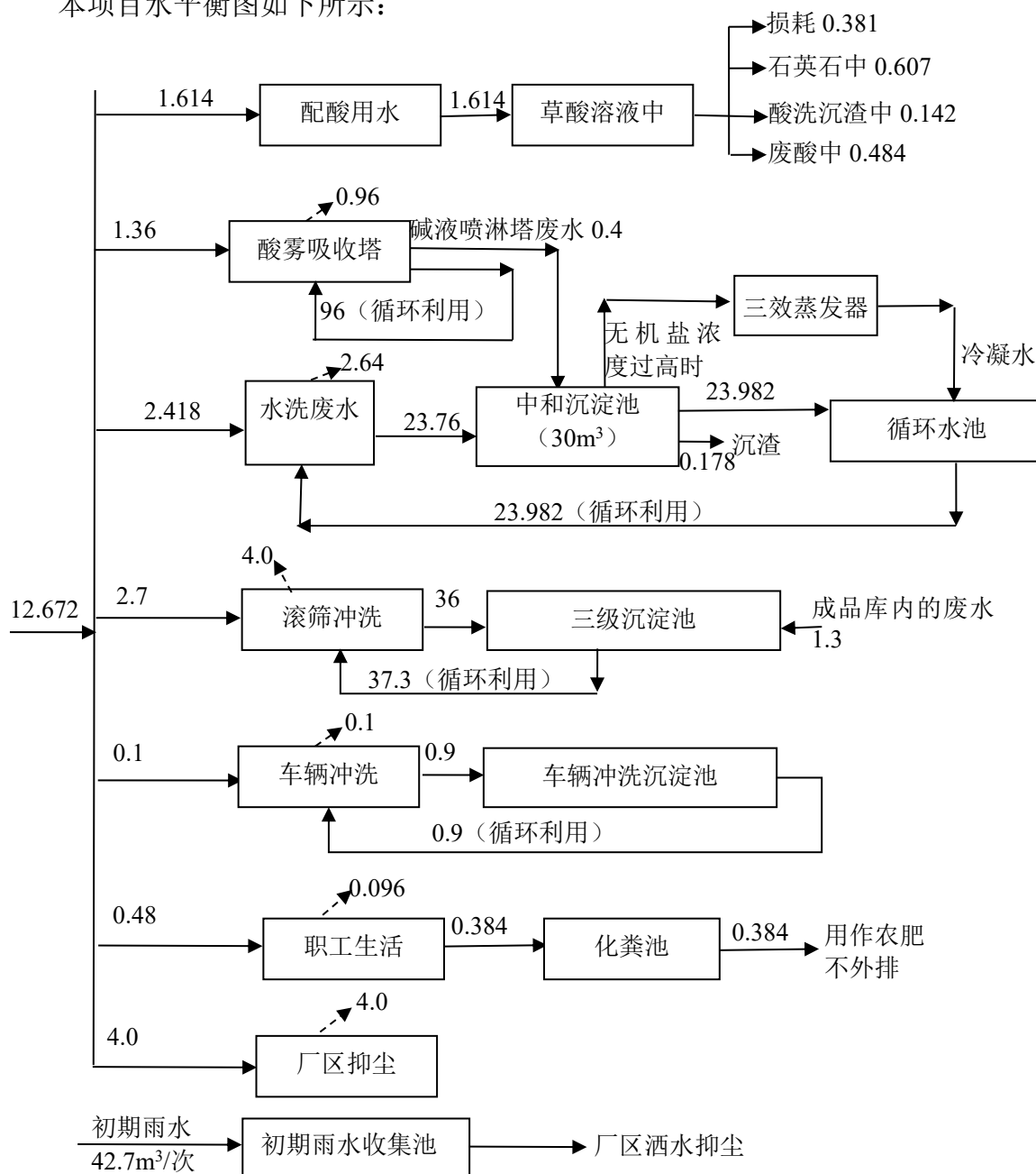
图 2-1 本项目日水平衡图 m³/d
