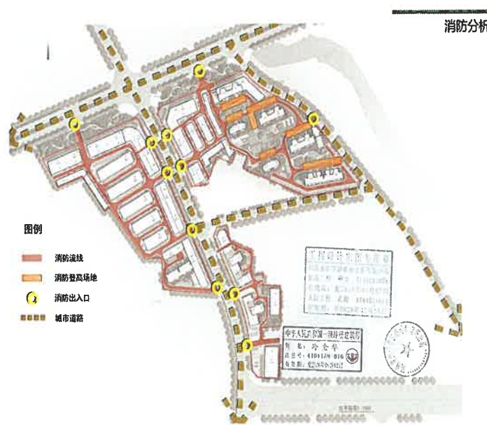
消防分析图
